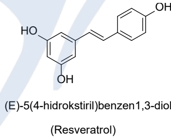
Şekil 1. Resveratrol Bileşiğinin Kimyasal Yapısı
