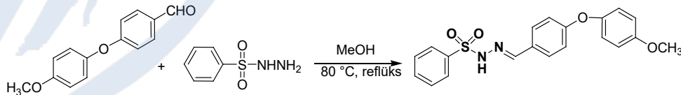
Şekil 1. N-Fenoksi aril sülfonil hidrazon bileşiğinin sentezi
